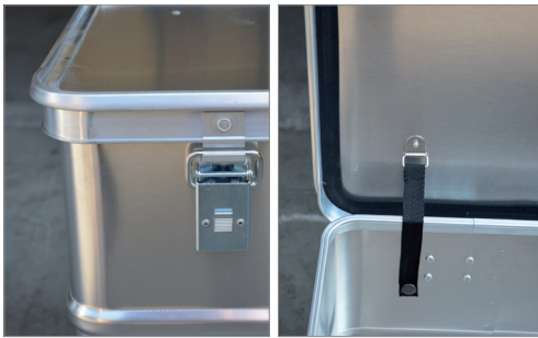
Hebelspannverschluss mit Aufspring-Sicherungsschnapper
